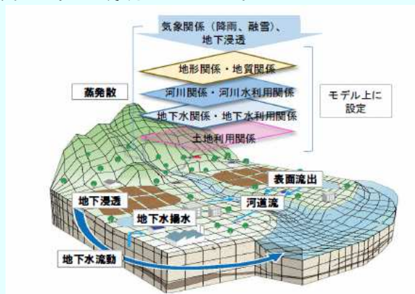
図の出典 「水循環解析に関する技術資料」 (国土技術政策総合研究所資料、第883号、H28.3)
