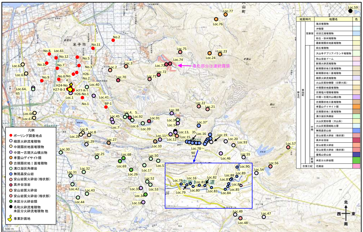
図3 地表地質踏査地点
