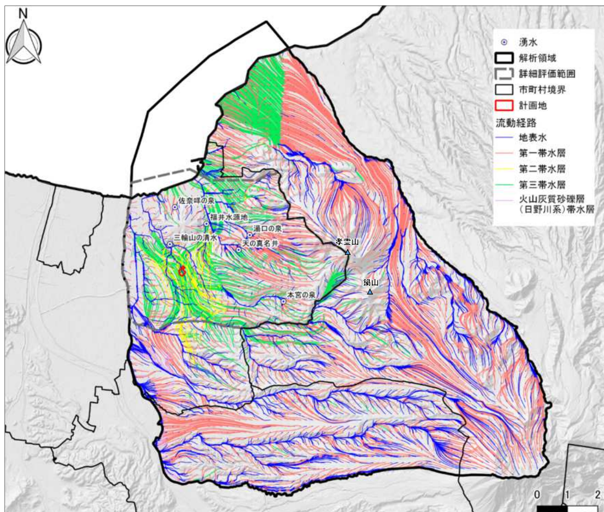
図24 流線図（広域）
