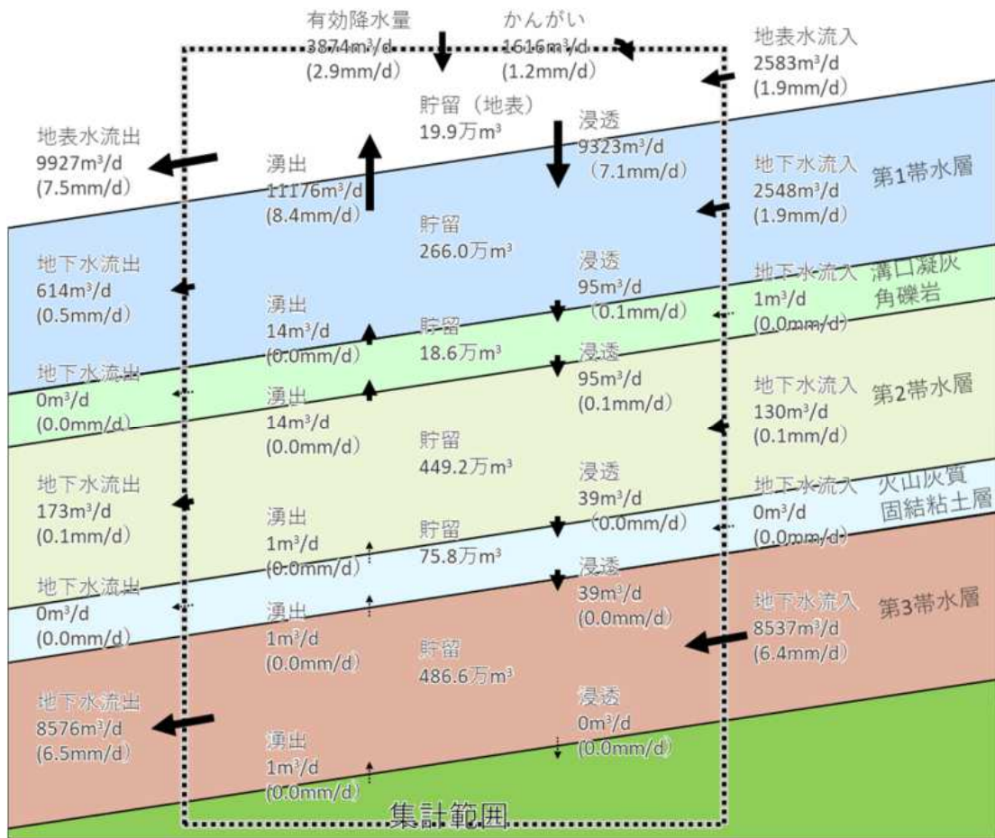
図27 水収支図
