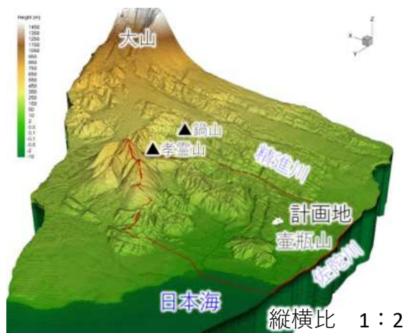
図20 3次元格子モデル
